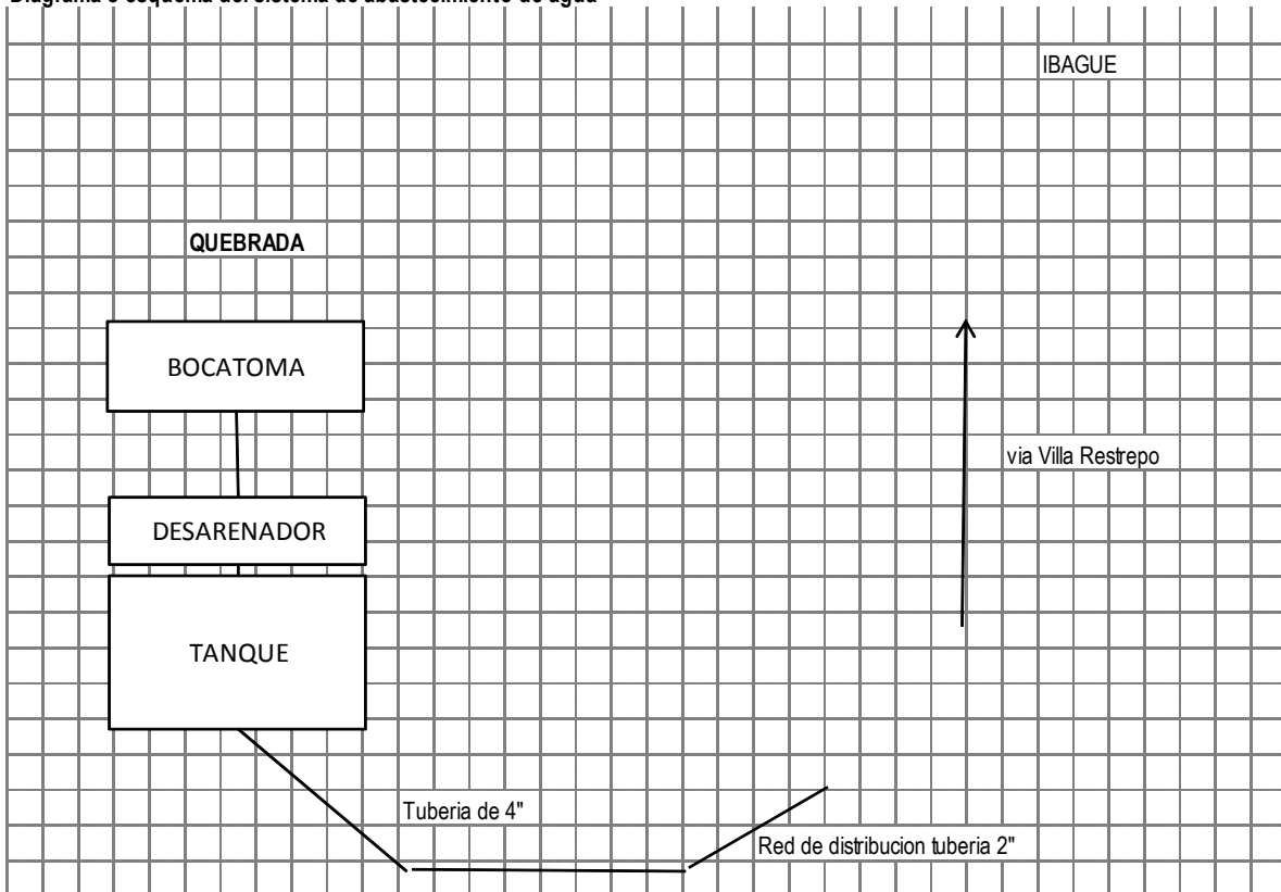
Diagrama o esquema del sistema de abastecimiento de agua
