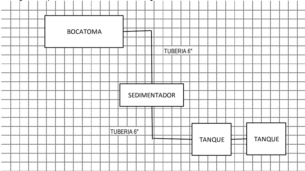
14. Diagrama o esquema del sistema de abastecimiento de agua
