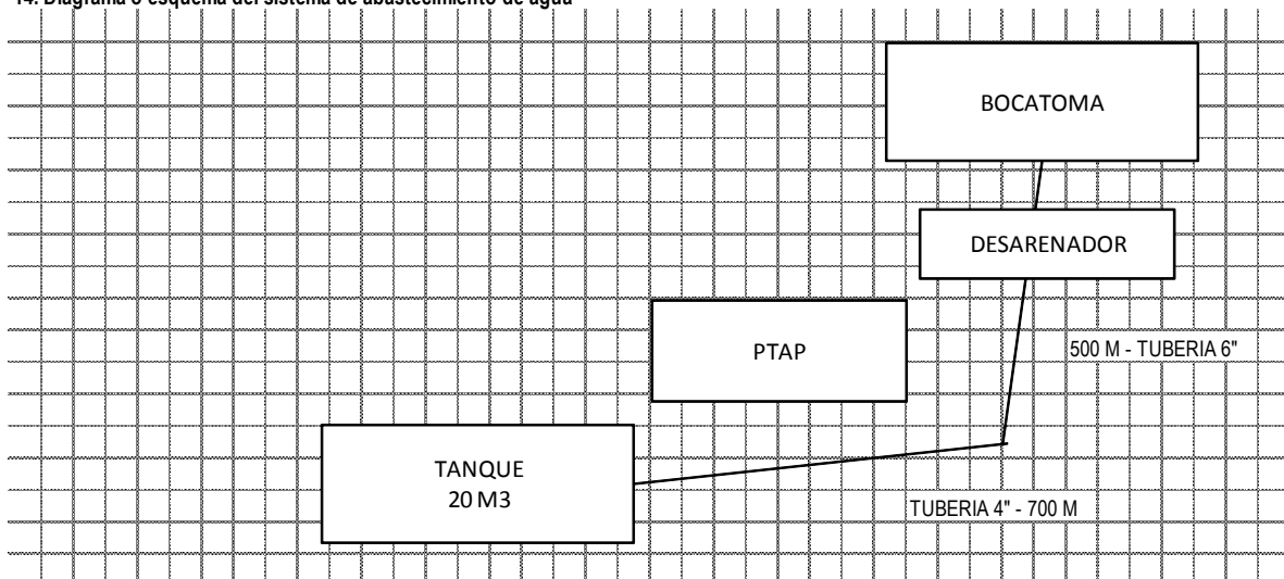
14. Diagrama o esquema del sistema de abastecimiento de agua
