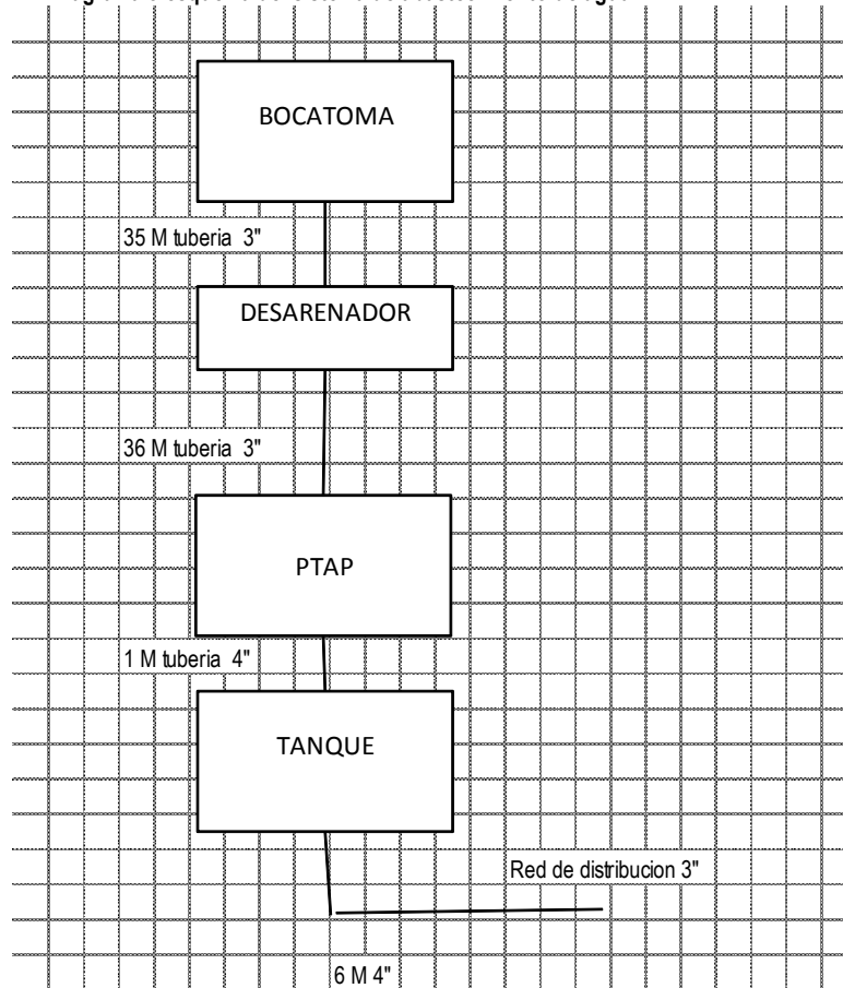
14. Diagrama o esquema del sistema de abastecimiento de agua
